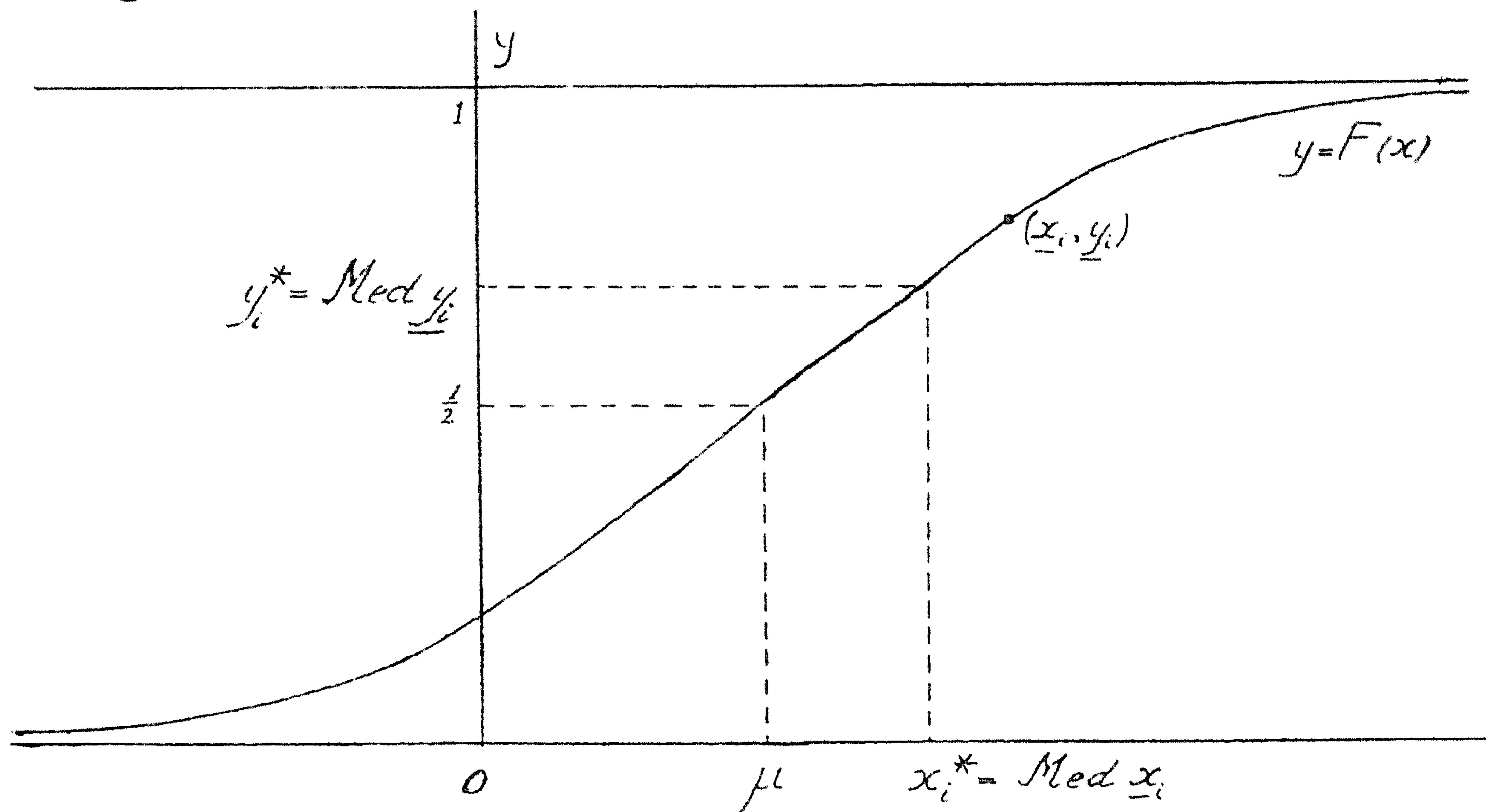
Fig. 1. Normale verdelingsfunctie op gewoon grafiekenpapier.
