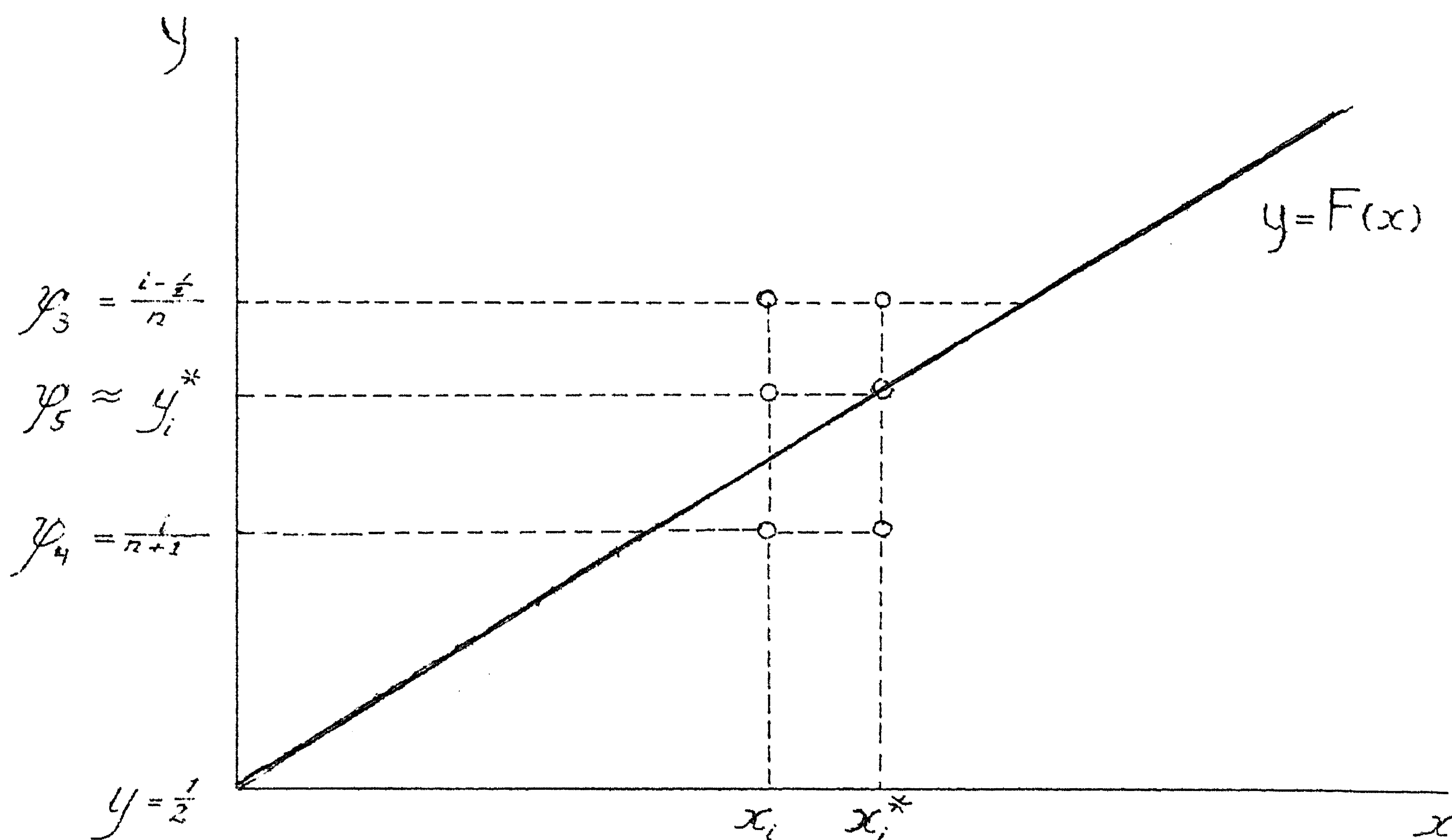
Fig. 2. Drie methoden voor het uitzetten van waarnemingen op waarschijnlijkheidspapier.
